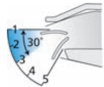
Im Kühlbetrieb wird die Luftleitlamelle stufenlos im oberen Bereich (zw. Pos. 1 und 3) geschwenkt.
